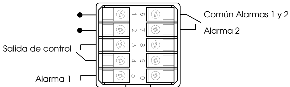
AK48 con 2 alarmas(las alarmas comparten un contacto común)
