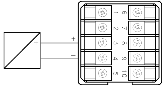
AK48: Salida para relé estático
