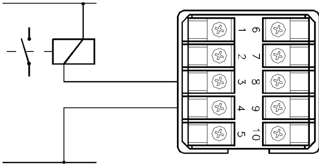
AK48: Salida para contactor
