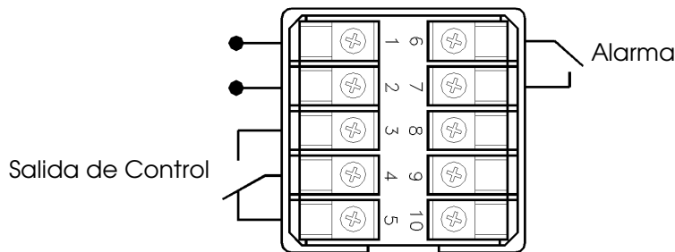
AK48 con 1 alarma
